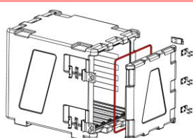
RR1027 Kit de juntas 5 ejemplares por paquete
