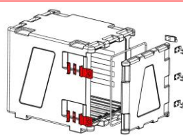
RR112 Kit de cierres completos 4 ejemplares por paquete
