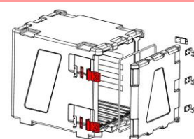
RR1004 Kit de cierres (sólo paleta) 4 ejemplares por paquete
